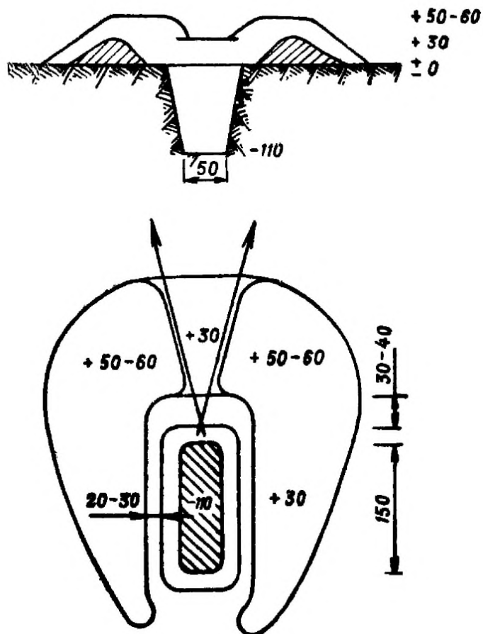
Одиночный окоп для стрельбы из автомата стоя
